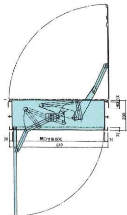
上ブタ下ブタ逆開閉避難口
