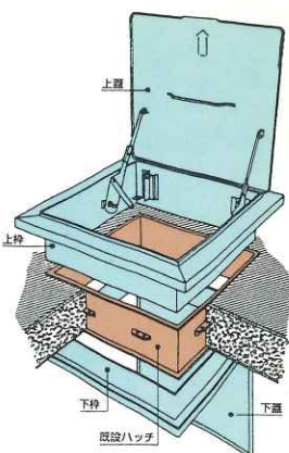
改修用避難口
