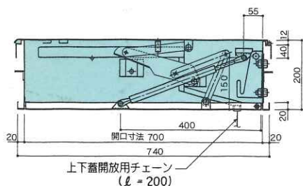
上・下階操作の避難口 (内寸600×600) (内寸700×700)
