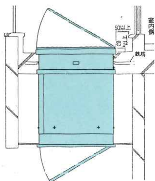
二重天井用避難口(胴長ハッチ)
